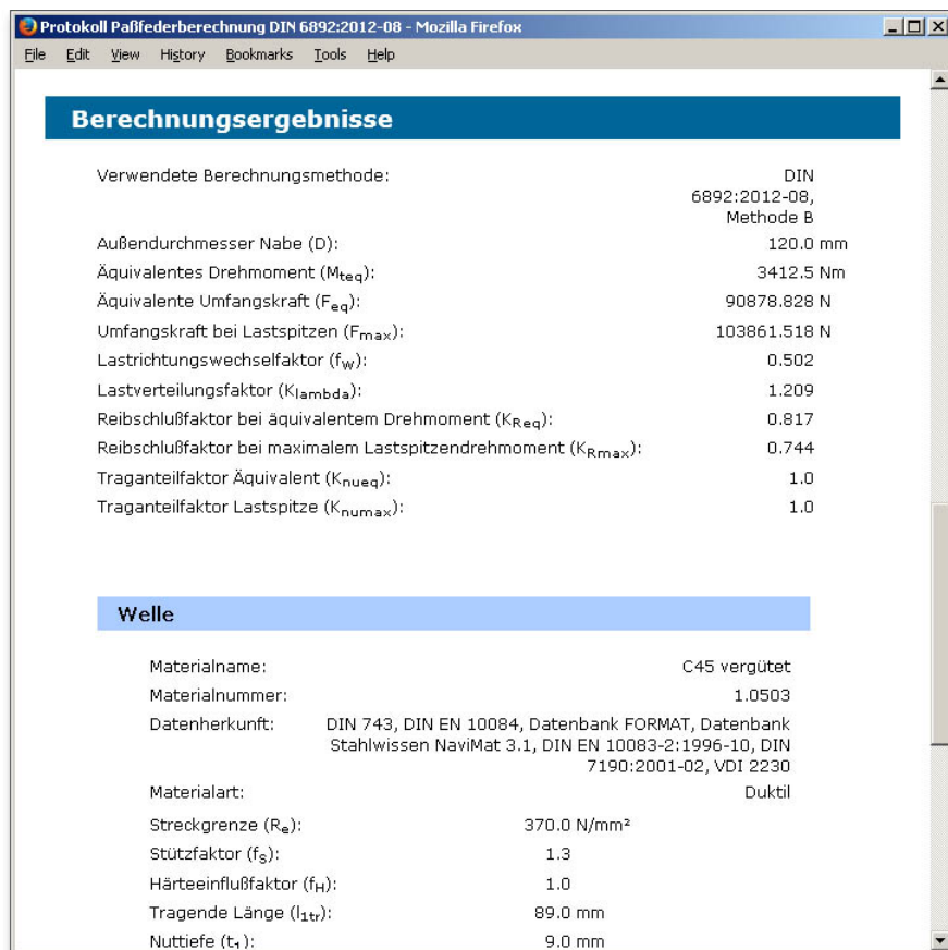
Abbildung 17: Berechnungsprotokoll
