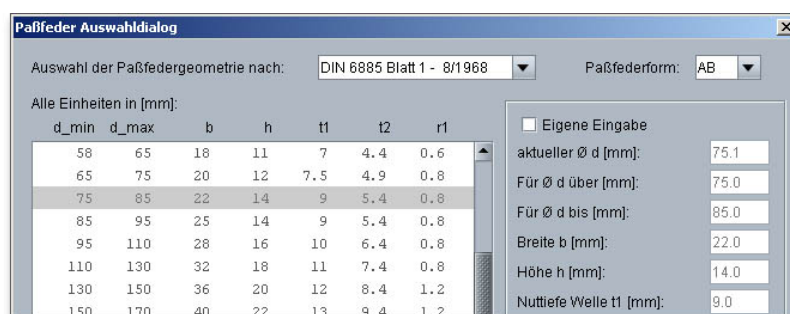
Abbildung 15: Neue Passfeder
